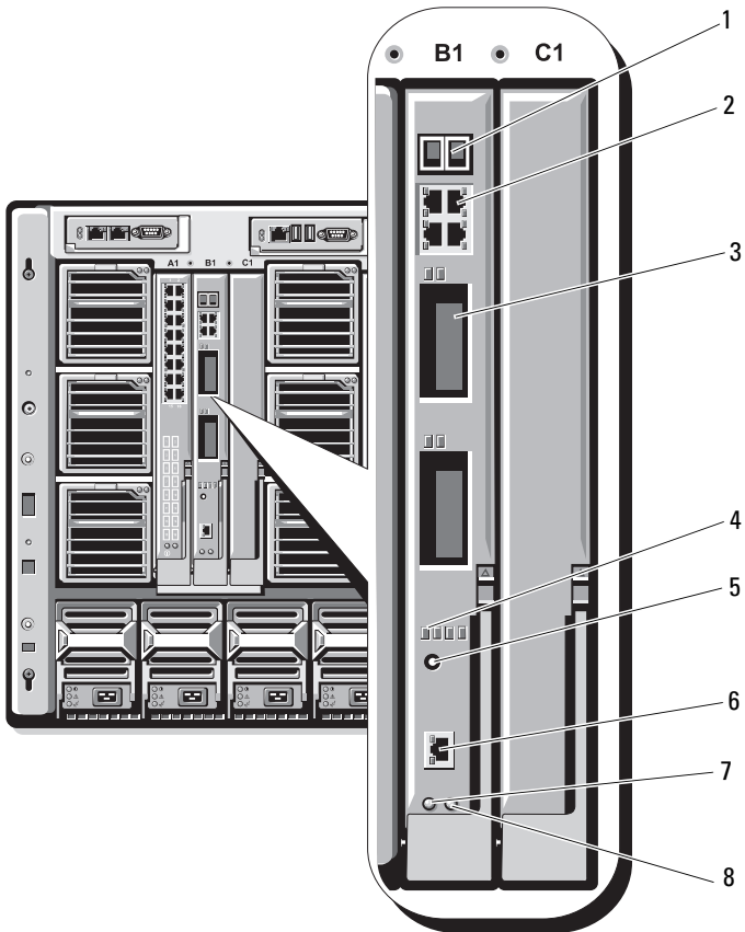
Figure 3-4. Fonctionnalités des modules commutateurs Ethernet Cisco
