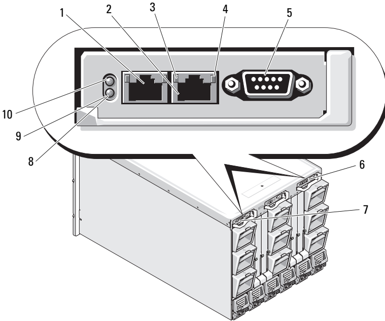
Figure 1-9. Fonctionnalités des modules CMC
